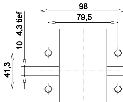
Maße - Getriebefuß
